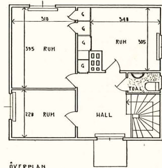
ÖVERPLAN
